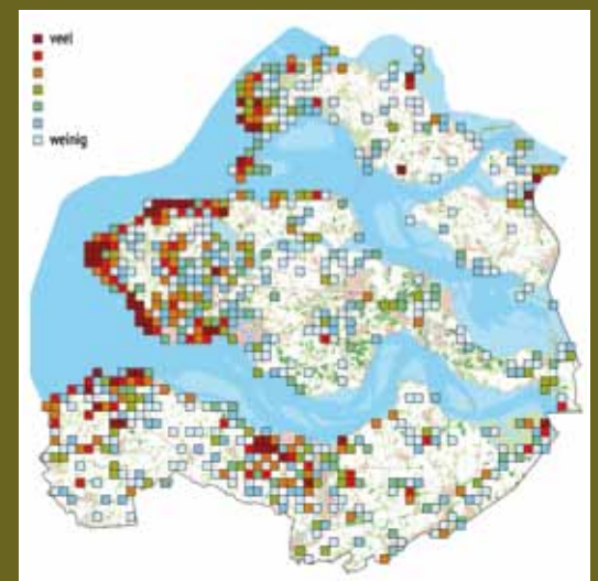
Beflijster: voorkomen per kilometerhok 1980-2020 (bron: Avifauna Zeelandica 2022)
