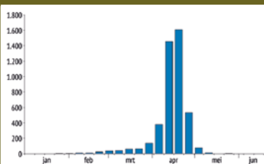
Graspieper - gemiddeld aantal per uur per standaardweek; Telpost Breskens in 1981-2020 (n=4.588.950, h=12.644) (bron: Avifauna Zeelandica 2022)
